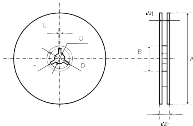
リール形状・寸法
