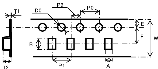
プラスチックテープ形状・寸法
