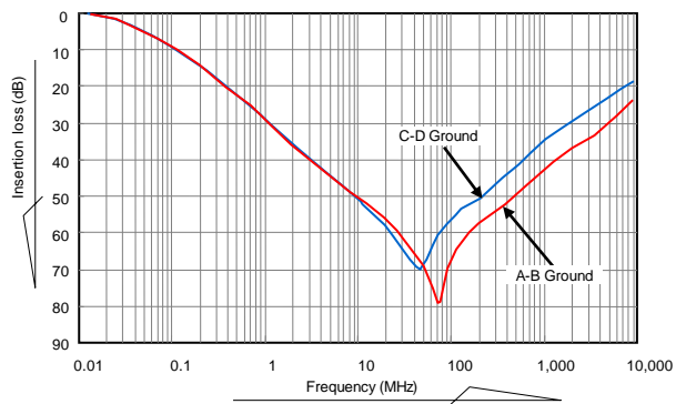
挿入損失特性(参考)
