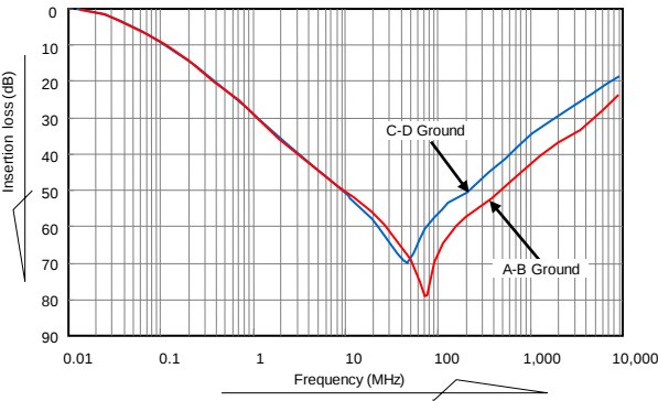
插入损耗特性（参考）
