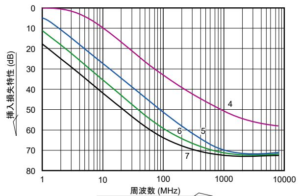
FTT40, FTT41型插入损耗特性数据
